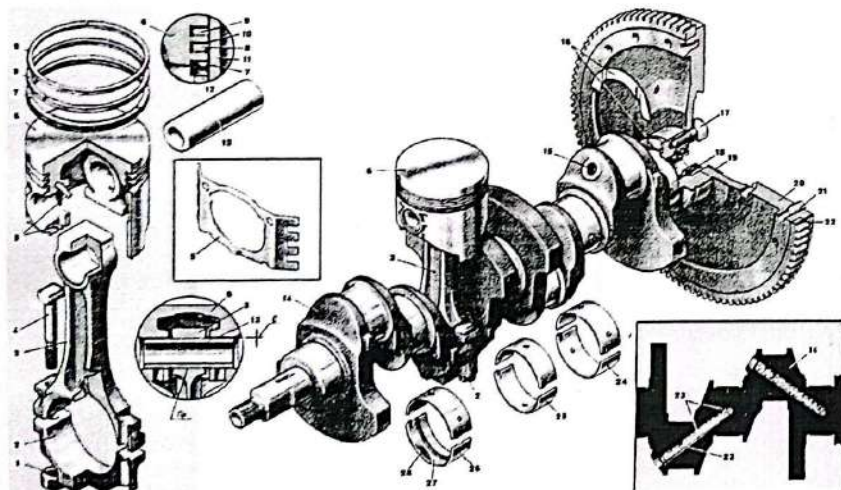
Krivoship shatunli mexanizmnin' uliwma korinisi
